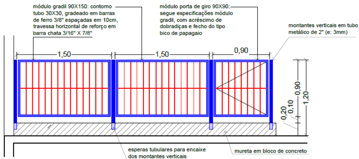
DETALHE GRADIL SUÍNOS Vista 1 escala: 1/25
