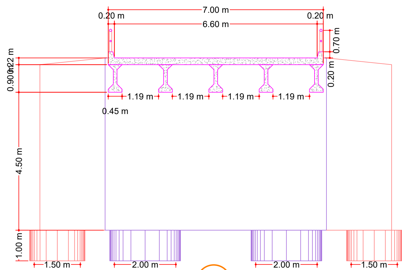
03 CORTE BB'
