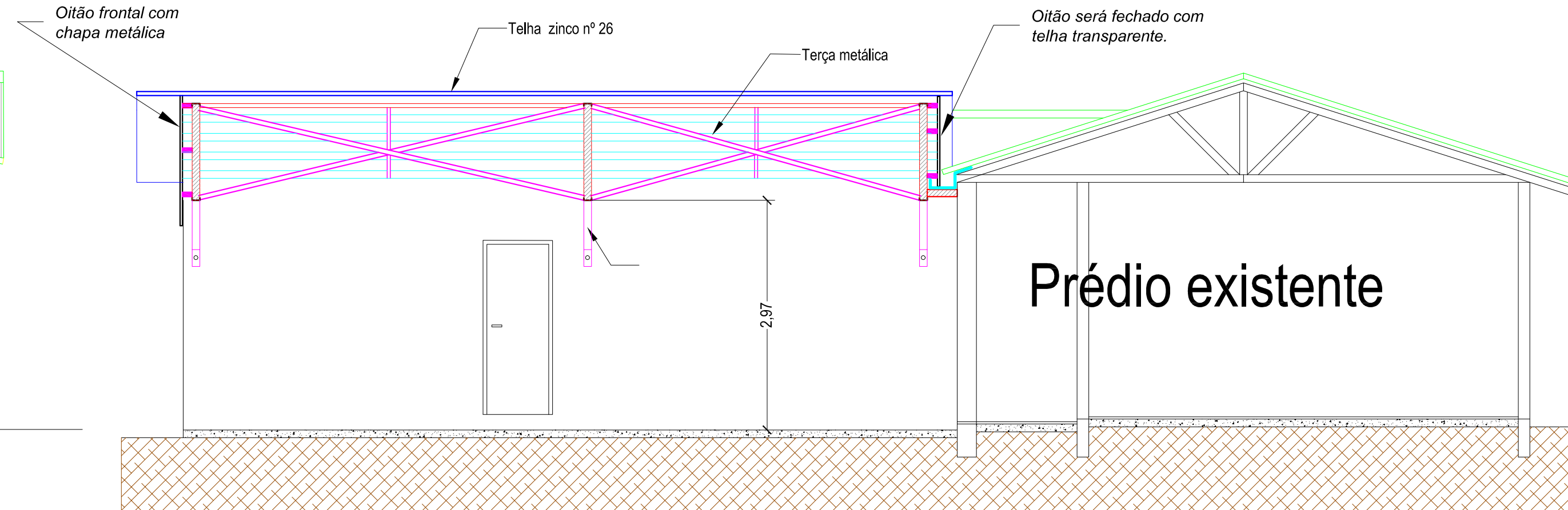
CORTE CD
