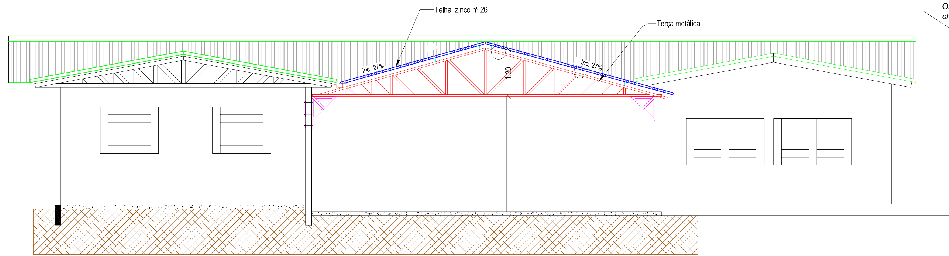
CORTE AB
