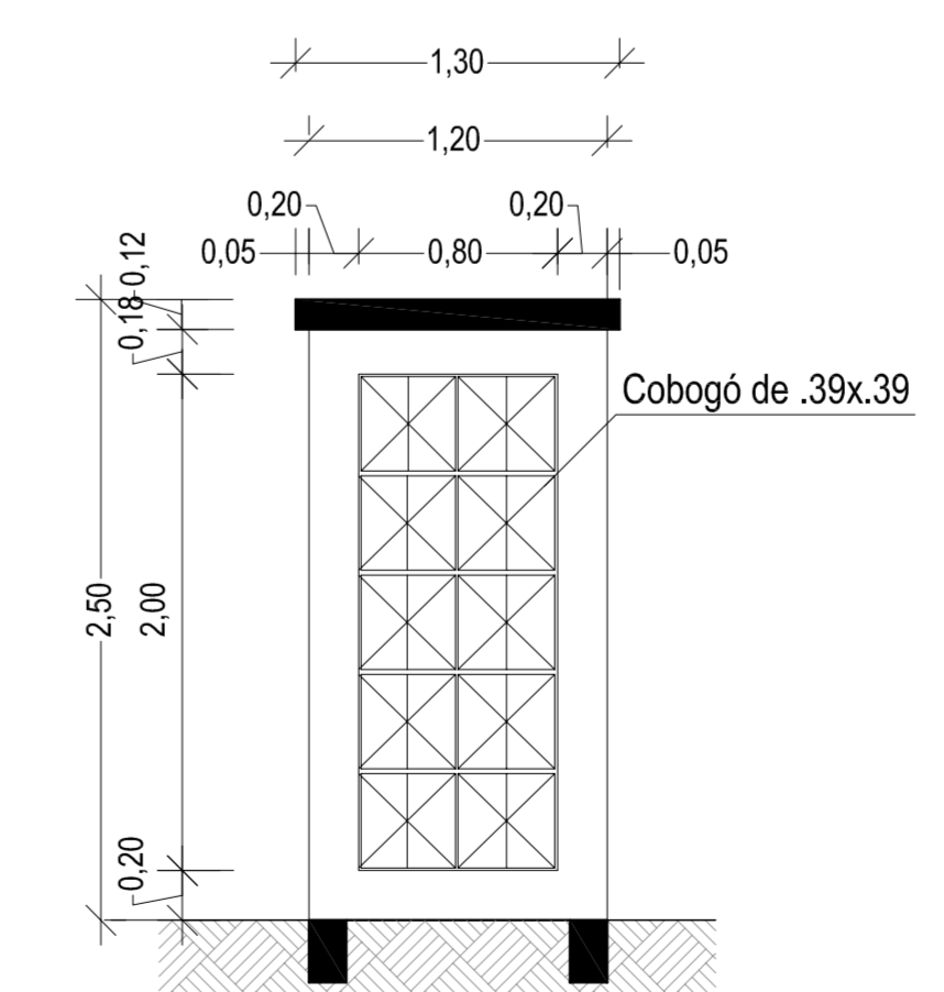
CORTE KL Escala 1/20
