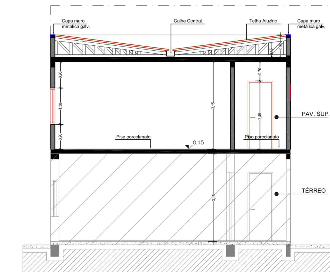
CORTE EF Escala 1/50
