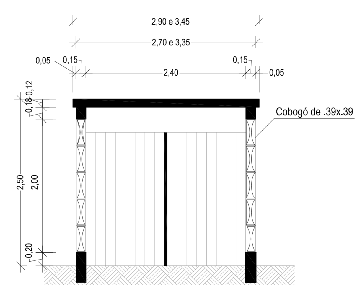
CORTE IJ Escala 1/20
