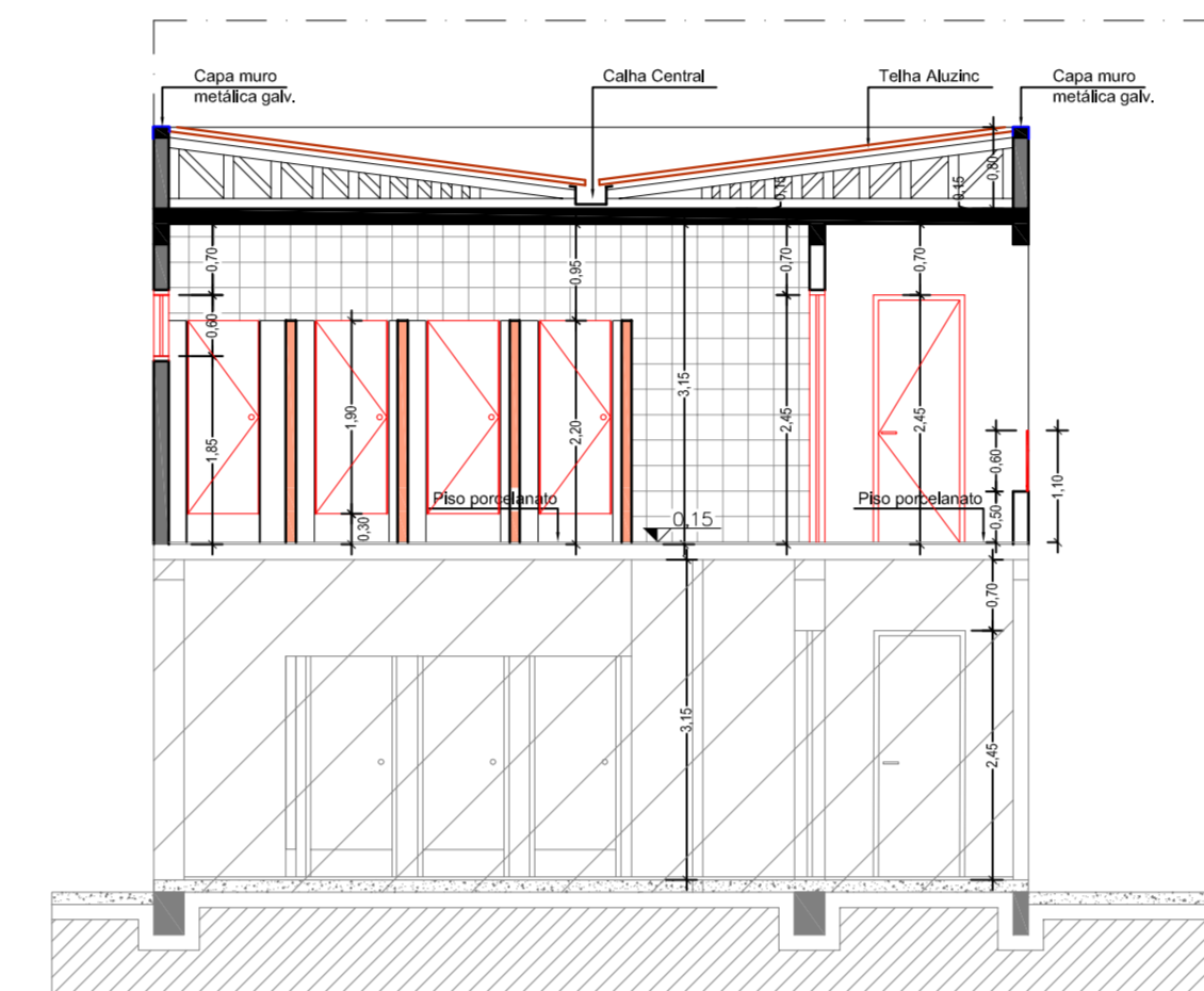
CORTE CD Escala 1/50
