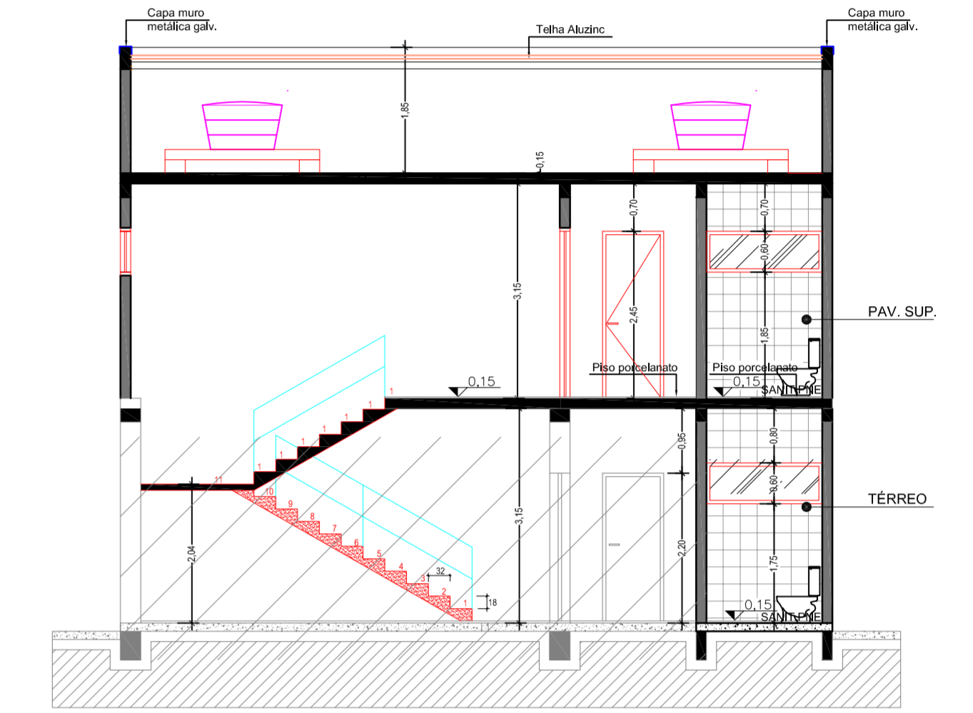
CORTE GH Escala 1/50
