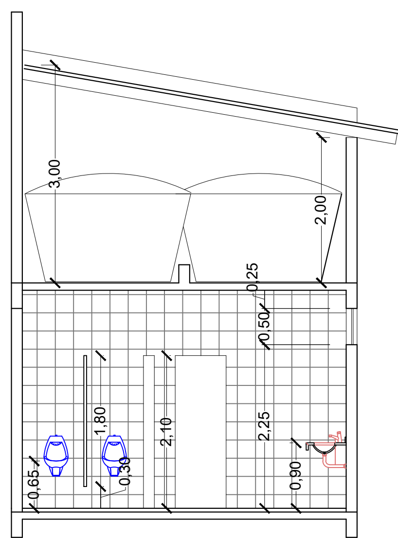
CORTE B B' Banheiros Pavilhão A
