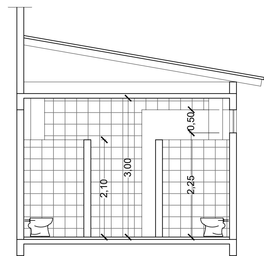
CORTE A A' Banheiros Pavilhão A
