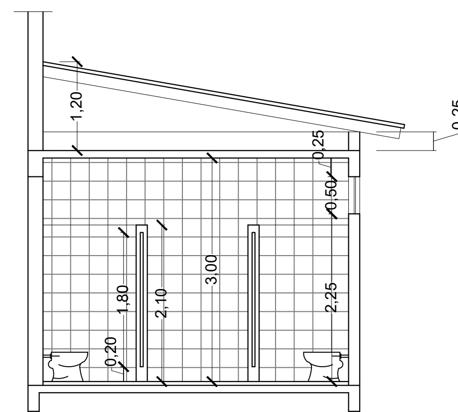
CORTE C C' Banheiros Pavilhão A
