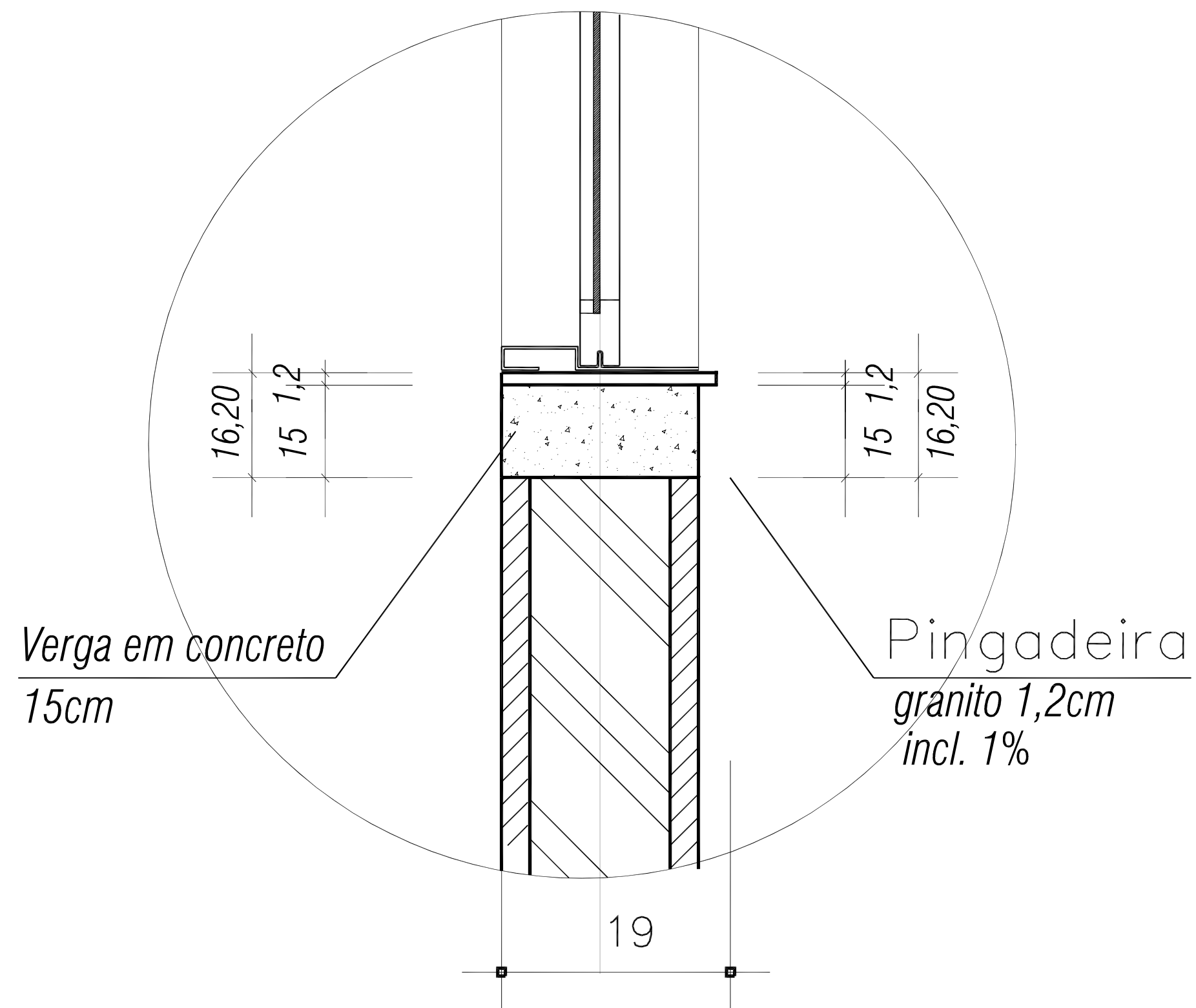
DET. SOLEIRAS DAS JANELAS – EM CORTE EXTERNA
