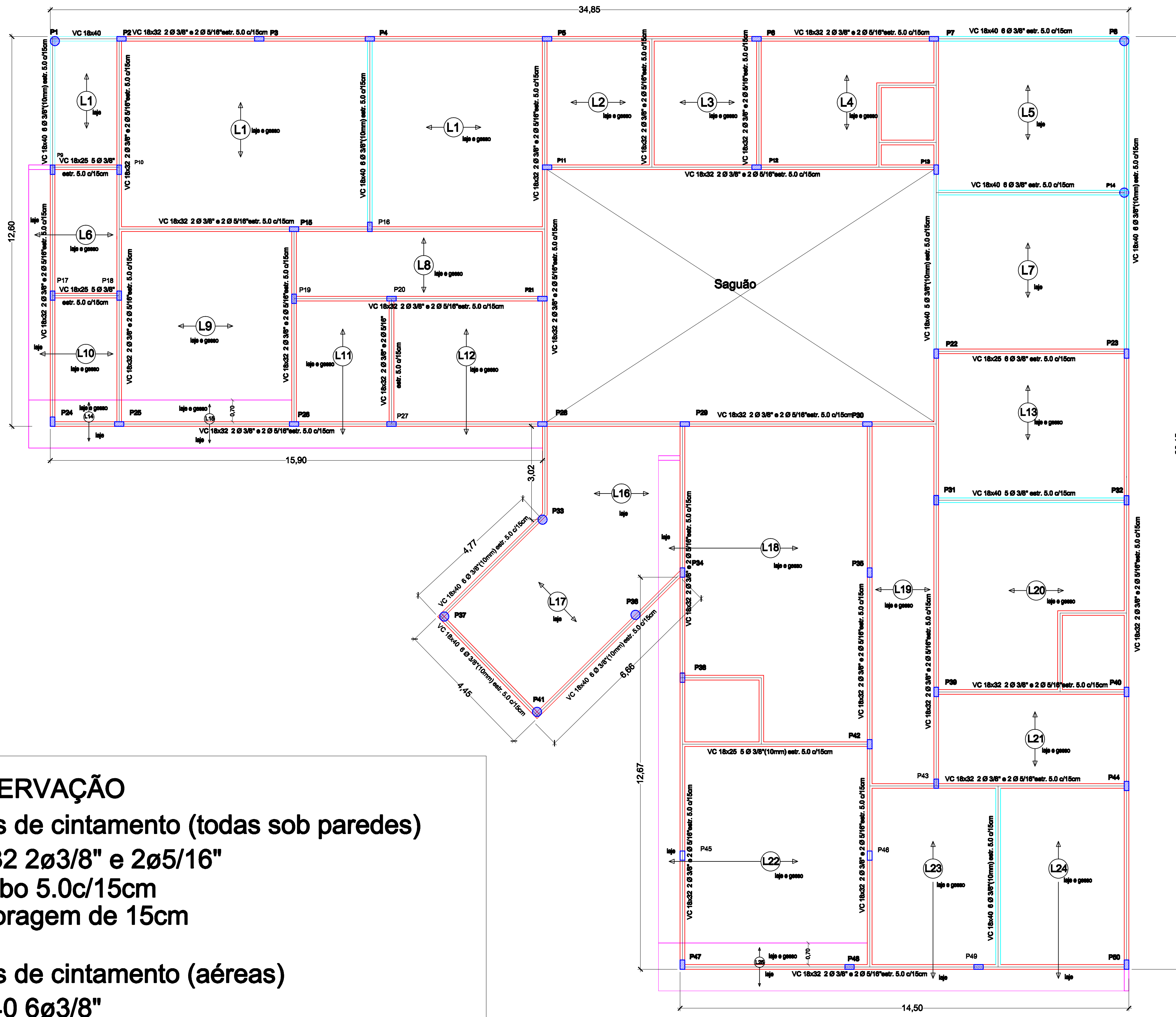
VIGA CINTAMENTO Cintamento, Pilares, laje Escala 1/75
