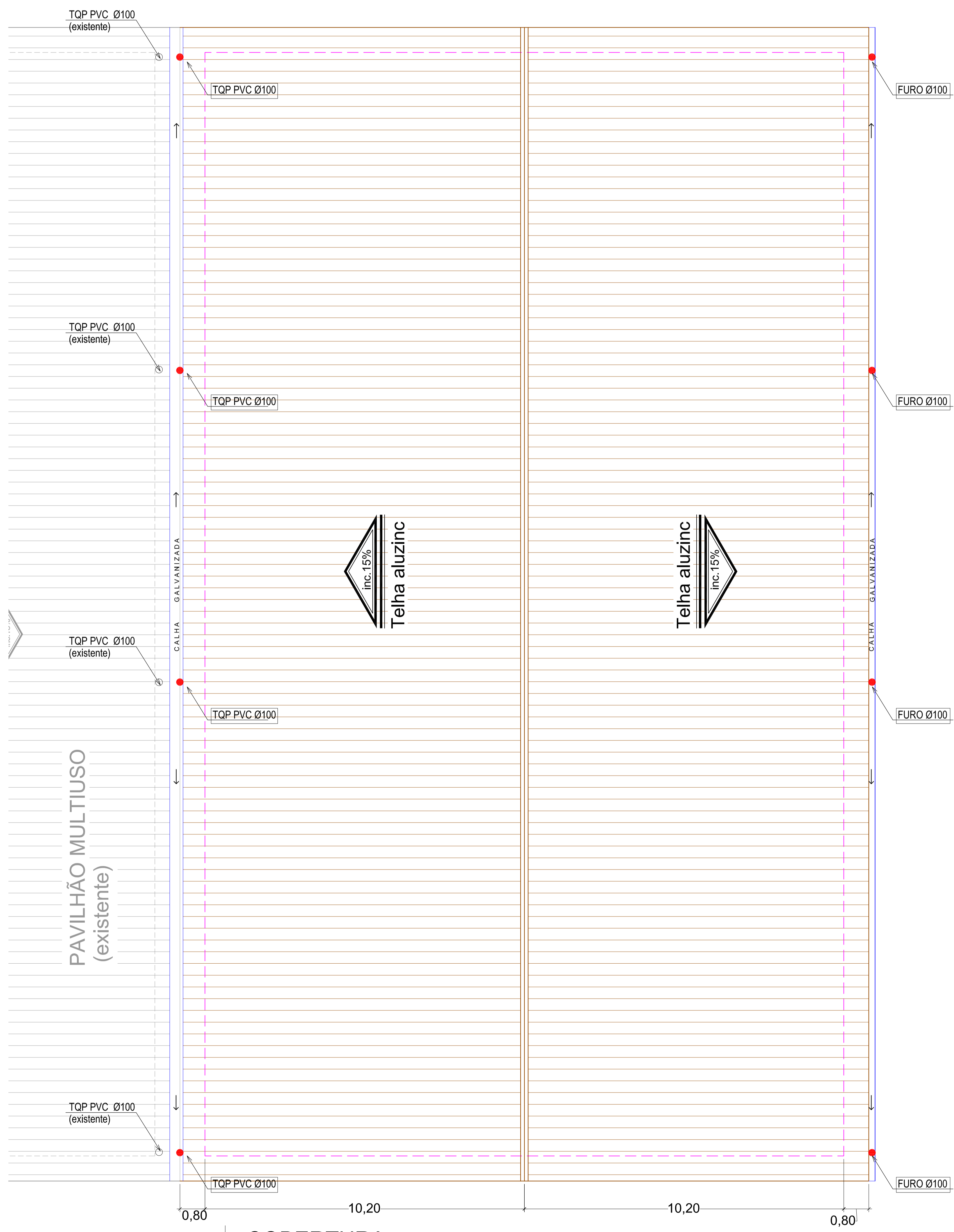
COBERTURA esc. 1/75
