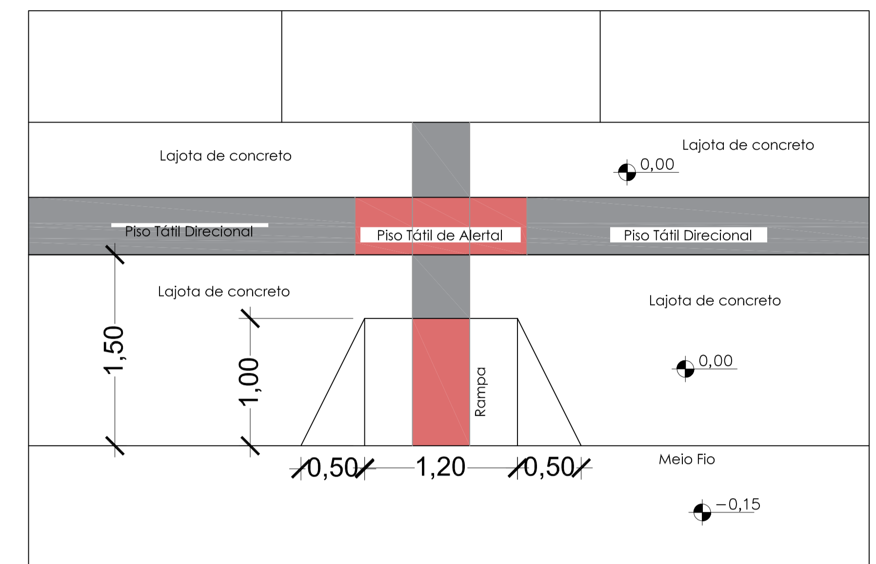
DETALHE RAMPA S/ ESCALA
