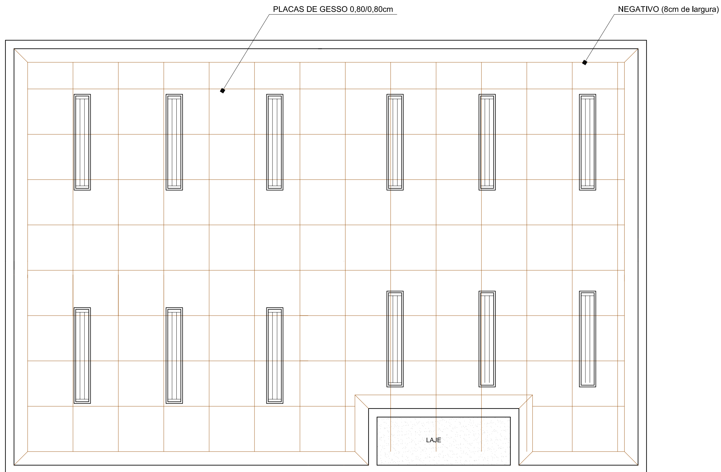
PLANTA DE FORMA-TODO O BLOCO escala 1/50
