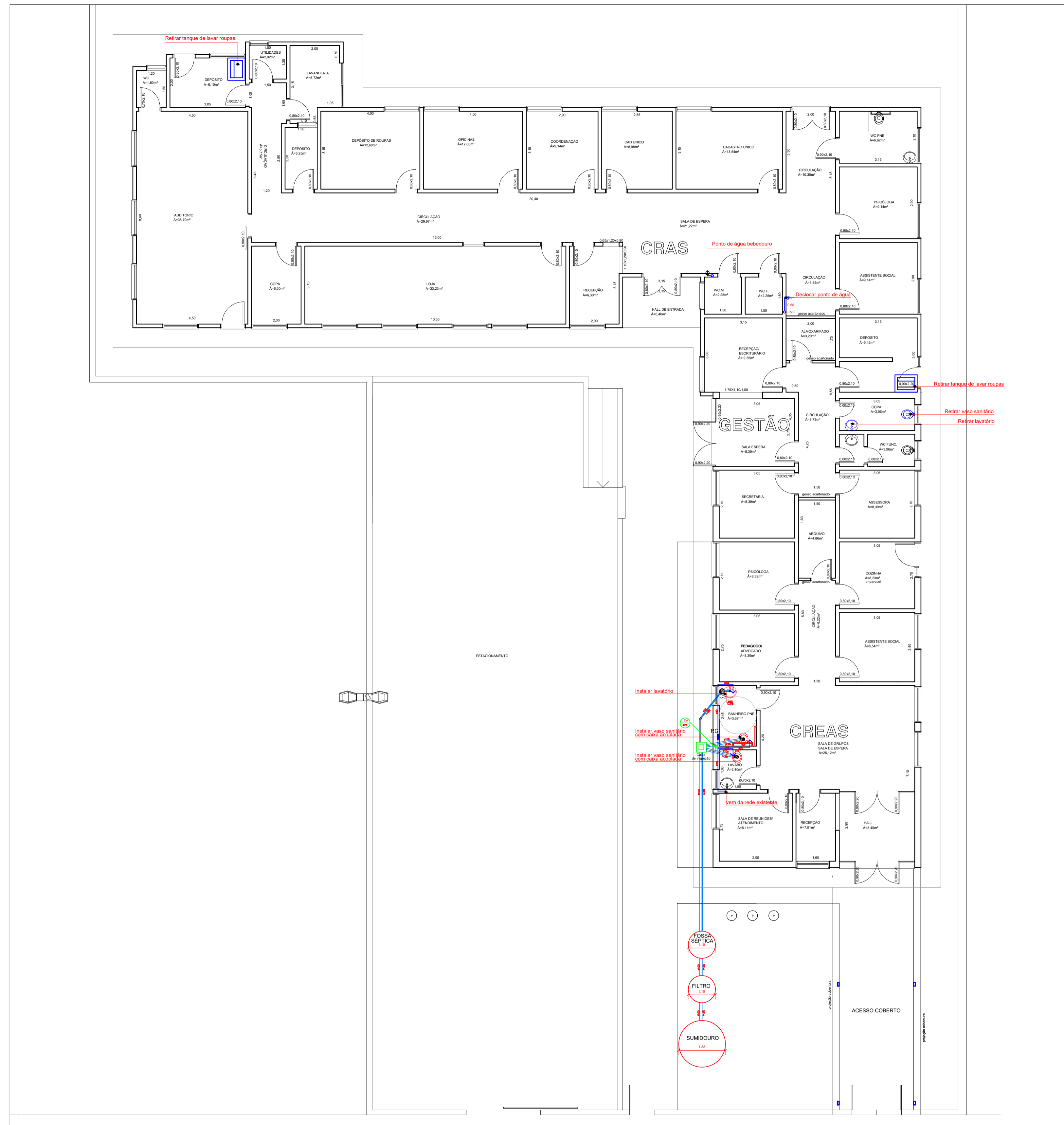
PLANTA BAIXA ÁGUA FRIA ESCALA 1/100
